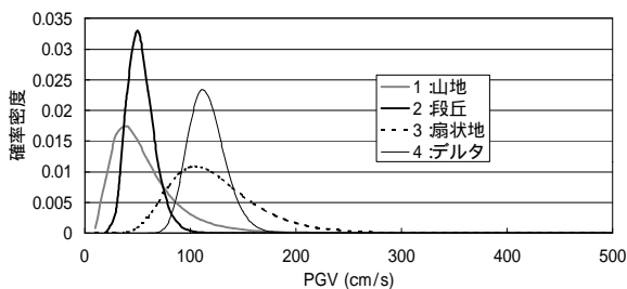
図 17 地盤ごとの PGV 生起確率密度分布関数
