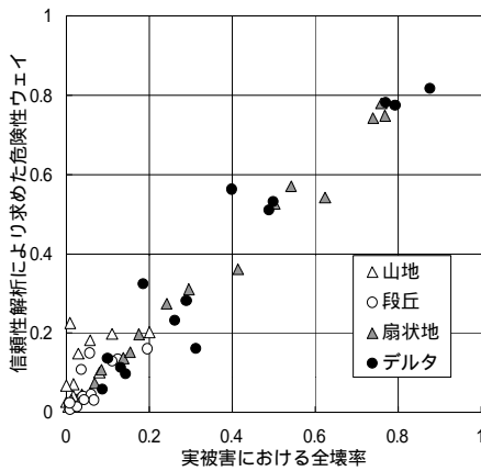
図19 危険性ウェイトの地盤ごとの再現性の評価
