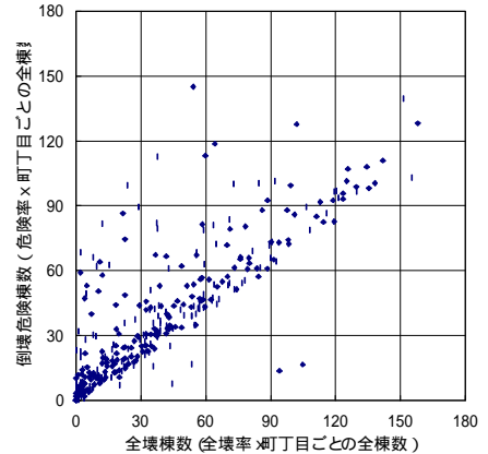
図15 全壊棟数と新建物危険棟数との比較
