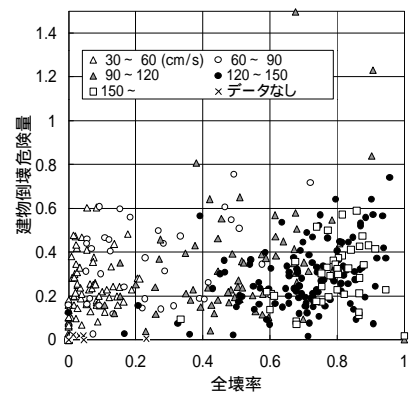
図9 全壊率と建物倒壊危険量の比較
